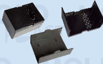
CÓD. 12143 PRETA -TAMPA CINZA MEDIDAS INTERNAS: COMP. 90MM LARG. 65MM ALT. 48MM
