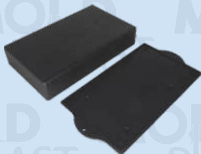
CÓD. 11326 PRETA MEDIDAS INTERNAS: COMP. 186MM LARG. 107MM ALT. 31MM C/ ABA
