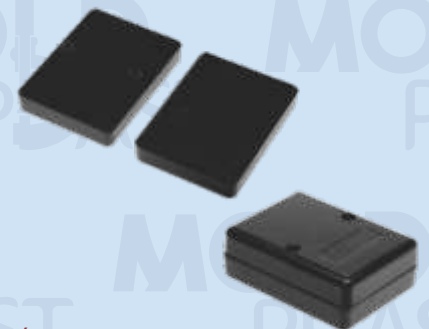
CÓD. 12164 MEDIDAS INTERNAS: COMP. 50MM X LARG. 36MM ALT. 15MM
