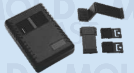
CÓD. 12522 CONTR. REMOTO 2 TECLAS CLIP BAIXO CÓD. 12533 CONTR. REMOTO 2 TECLAS CLIP ALTO MEDIDAS INTERNAS: COMP. 80MM X LARG. 55MM ALT. 15MM
