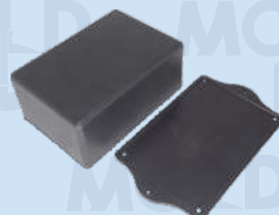
CÓD. 11138 PRETA MEDIDAS INTERNAS: COMP. 117MM LARG. 78MM ALT. 45MM - C/ ABA
