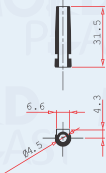
CÓD. 2875 DESCRIÇÃO: PASSO CABO AVULSO APLICAÇÃO: CABOS PARA FONTES DIV.
