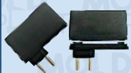
CÓD. 11173 PRETO C/ PINO VERTICAL MEDIDAS INTERNAS: COMP. 83MM LARG. 24MM ALT. 47MM
