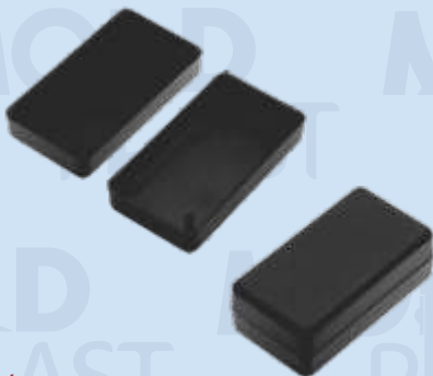
CÓD. 12162 BALOON MEDIDAS INTERNAS: COMP. 47MM X L.24MM ALT. 14MM
