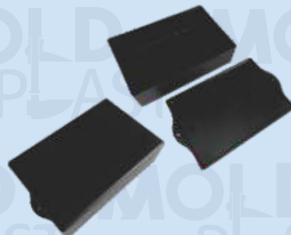
CÓD. 11644 PRETA MEDIDAS INTERNAS: COMP. 142MM LARG. 92MM ALT. 38MM C/ ABA
